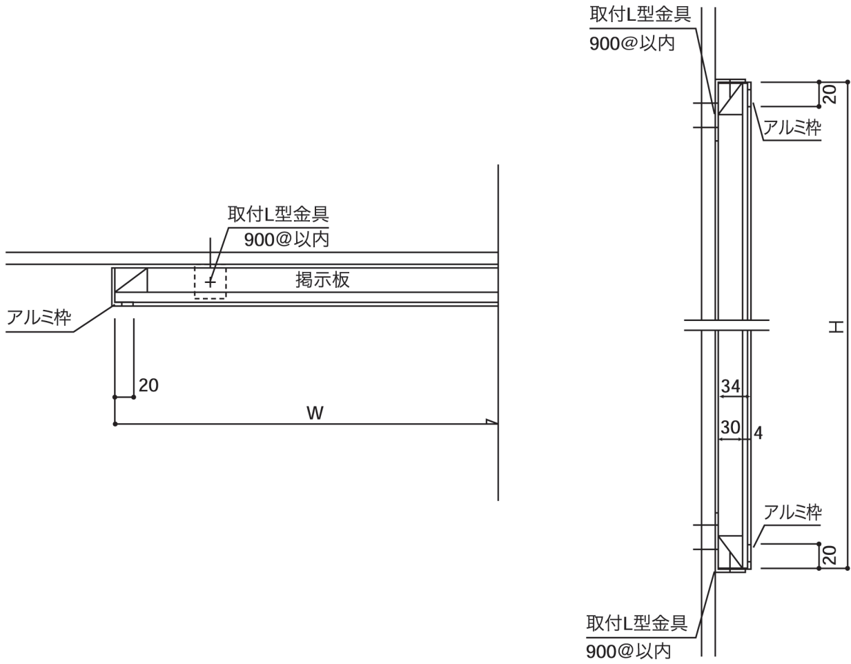
大型掲示板詳細図
