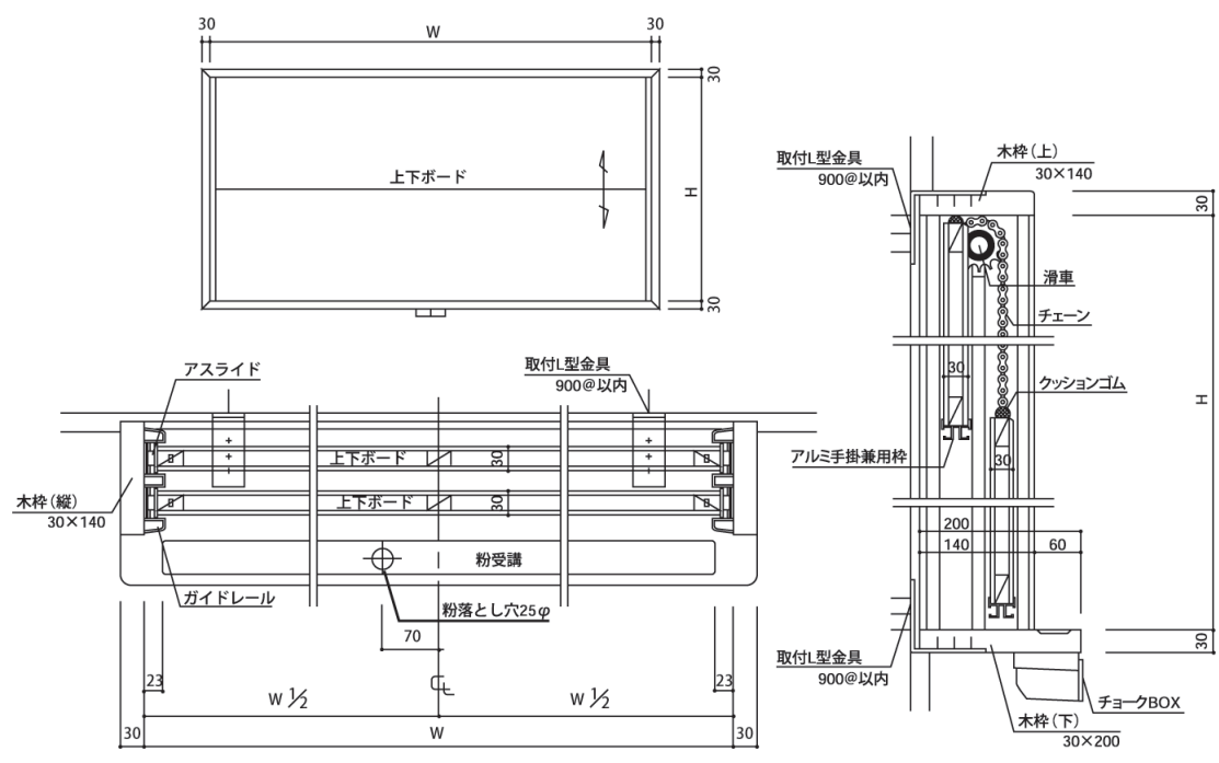
詳細図 (木枠付き)
