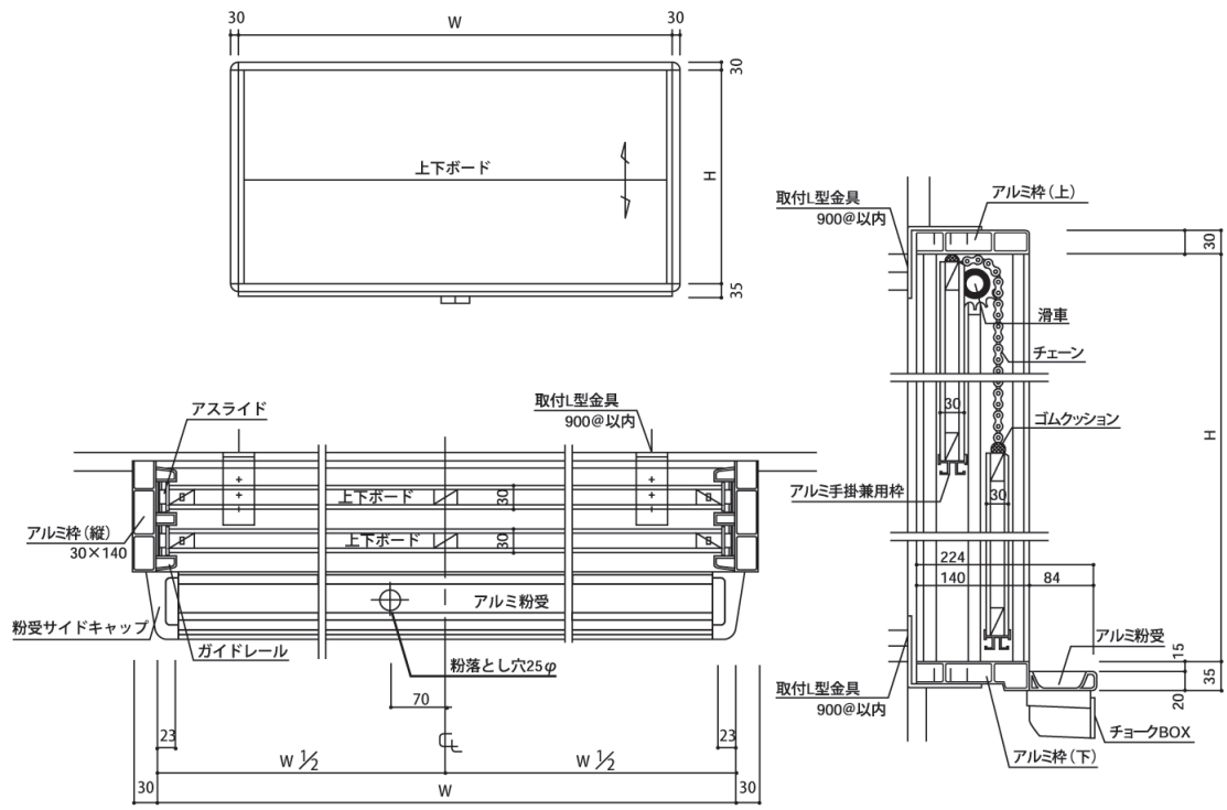
詳細図 (アルミ枠付き)
