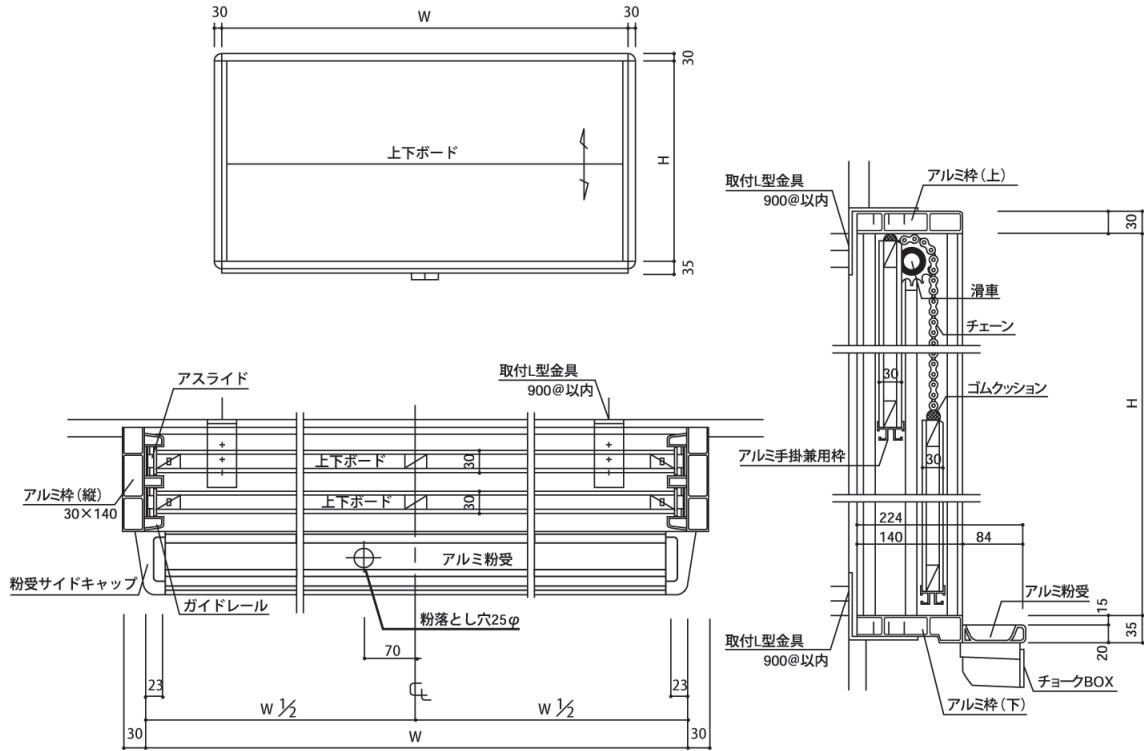
アルミ枠上下ボード詳細図
