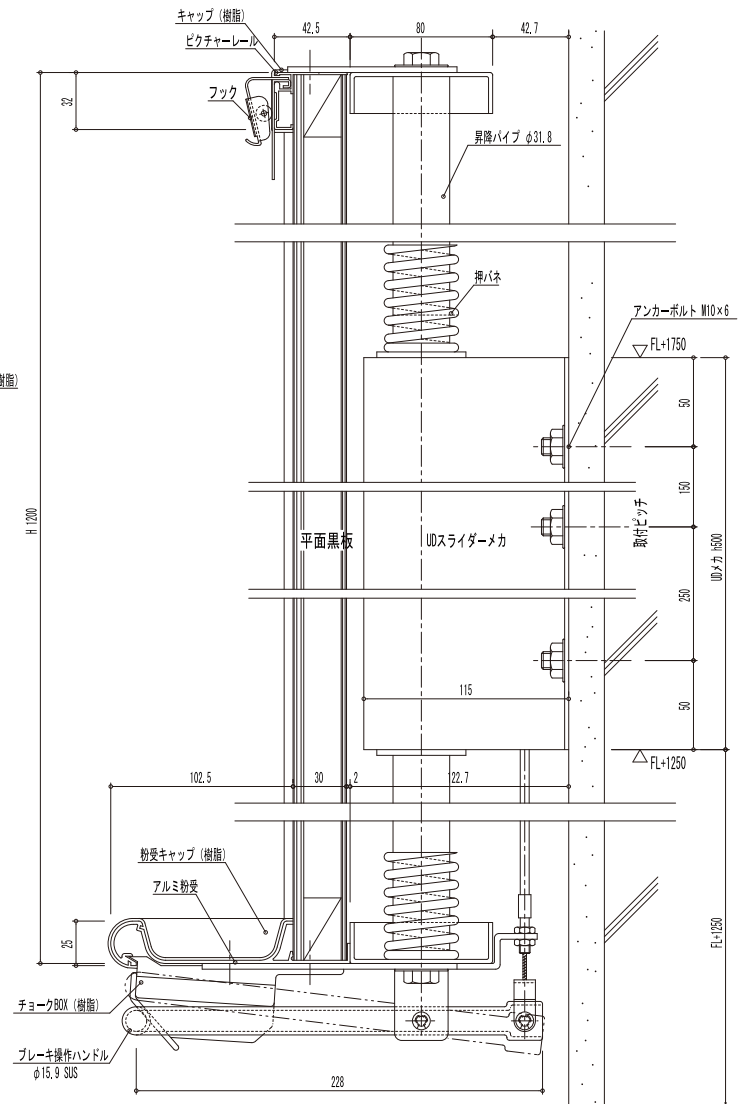
縦断面図
