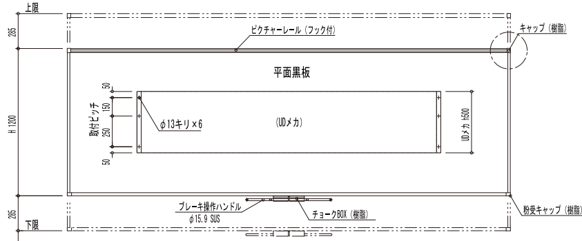
展開図
