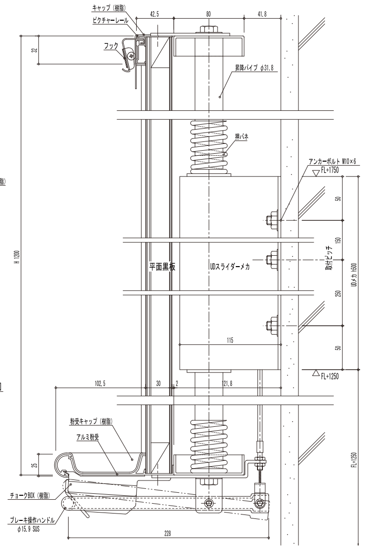
縦断面図
